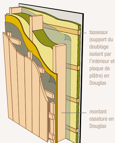
SOLUTION 2 : Structure primaire avec doublage isolant intérieur
